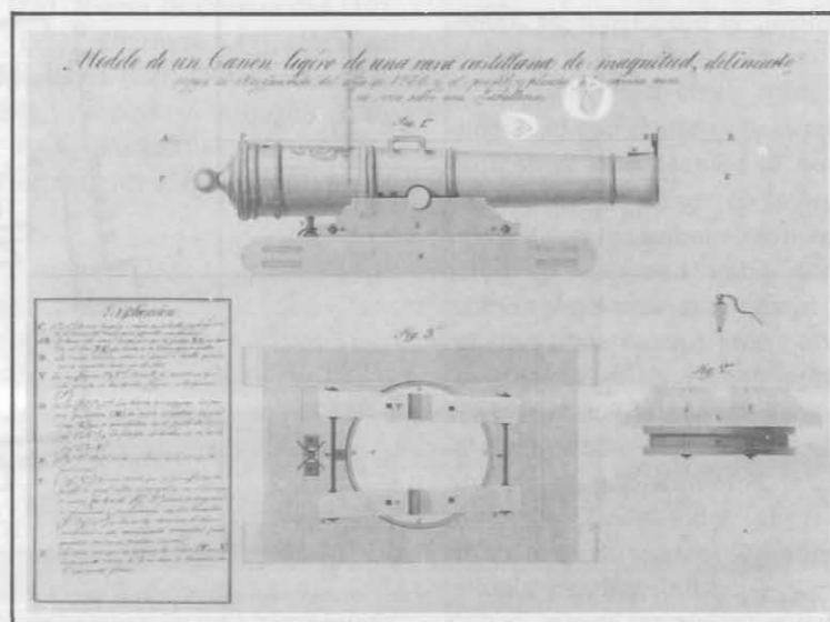
Cañón ligero de una vara castellana de magnitud, por Nicolás Ibañez, 1817. Indiferente de Guerra, vol. 201, f. 215 (3 338).
