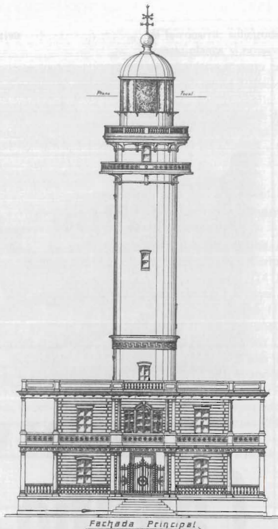
Proyecto de faro para Coatzacoalcos, México, 1911. Comunicaciones y Obras Públicas, Anales de la Secretaría de Comunicaciones y Obras Públicas, núm. 7, lám. 11 (detalle).
