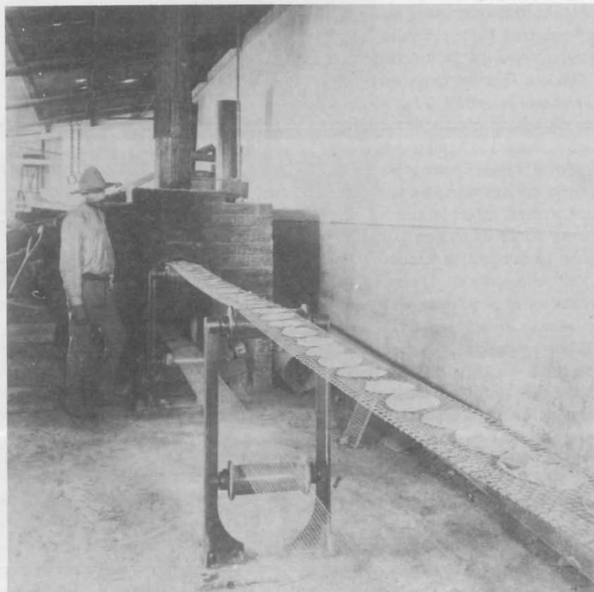
Máquina para hacer tortillas, México. Luis Romero Soto, vol. 1, sobre 10.
